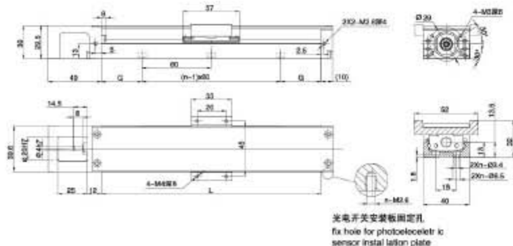
GSX40 电机连接器 Motor socket
